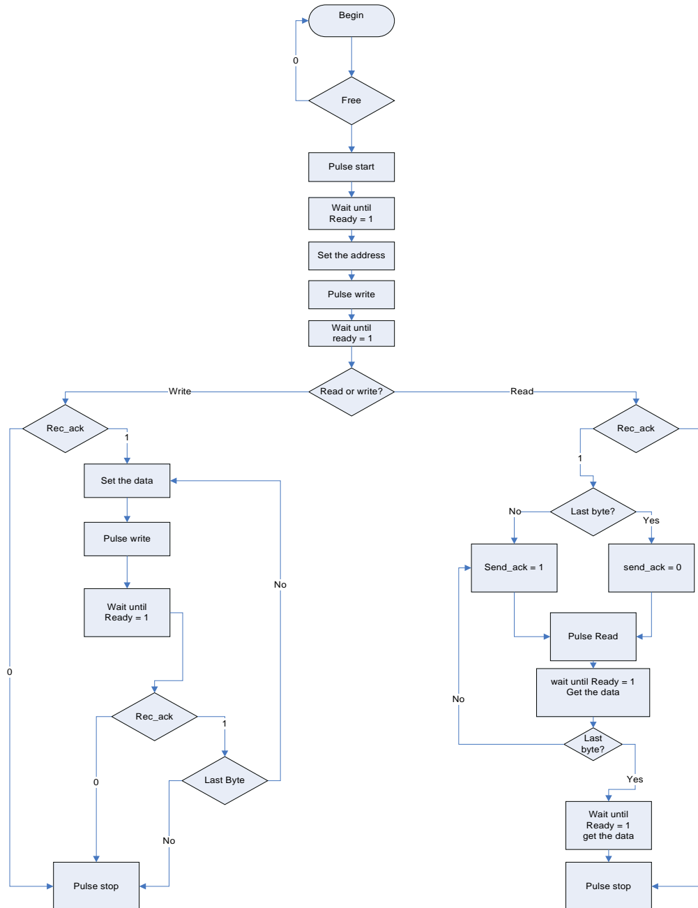
איור 10 תרשים זרימה להפעלת בקר I2C
