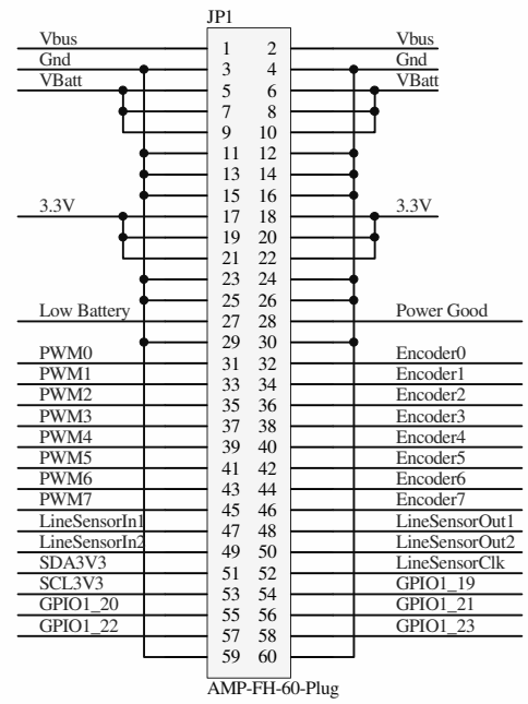
AMP-FH-60-Plug
