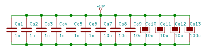
Capacitores bypass para VCC_AUX.
