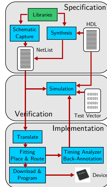
Fig. 6. Flujo de diseño usando HDL.
